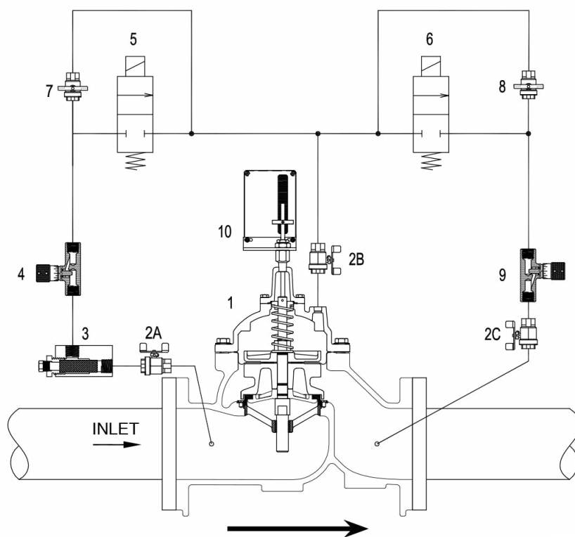
FIG. 2 Schematic A-7637A
