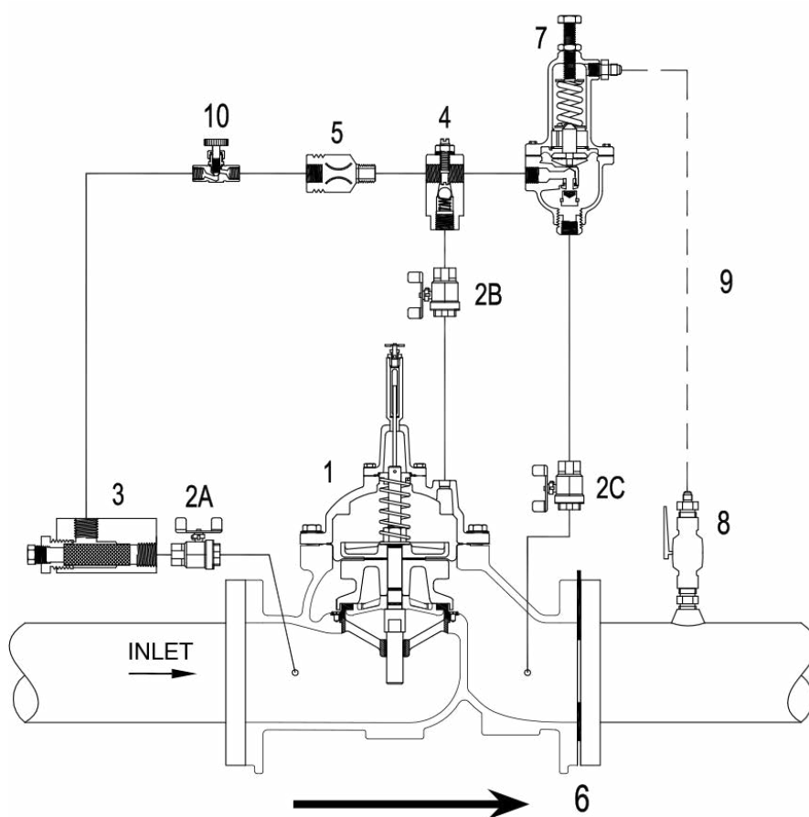
FIG. 2 Schematic A-7427C
